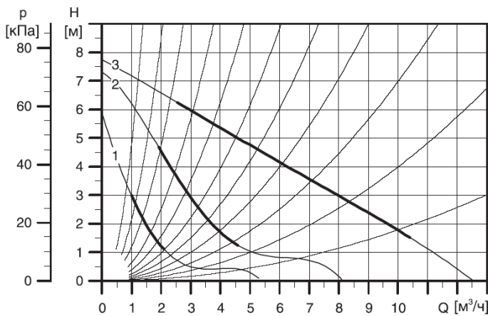
GRUNDFOS UPS 32 – 80
